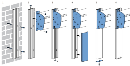
fig. 1.4 Montage van muurstrip (links)
