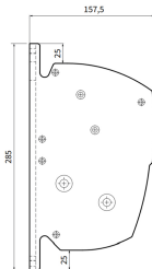
zijzicht muursteun links
