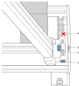
fig. 4.1 Detail armverbinding rechts
